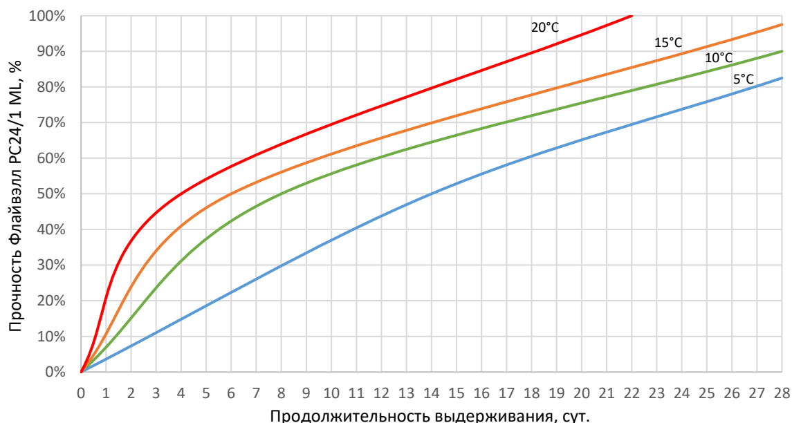
Рис.1. Прочность цементной штукатурки Флайвэлл РС24/1 ML в зависимости от температуры и продолжительности выдерживания.
